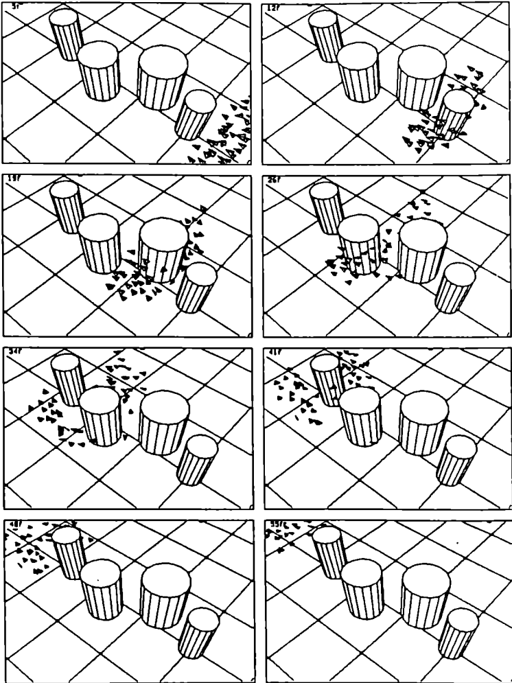
Figure 5. Un vol de boids . Dès lors que le comportement du groupe émerge des interactions locales individuelles de chaque boïd , on ne peut prédire à l'avance comment le groupe réagira face à un obstacle. Ici, la volée se sépare temporairement en deux pour fusionner à nouveau après les obstacles
