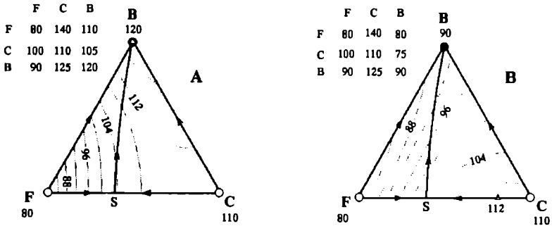
Figure 3. Flux des fréquences des stratégies et gradient de la fitness moyenne dans le jeu Faucon-Colombe-Bourgeois (o : point de fuite ; • : attracteur ; S : point-selle). (A) Jeu original (d'après Maynard Smith) : la fitness moyenne maximale est atteinte pour une population composée de 100 % de Bourgeois (SES). (B) Dynamique du jeu quand on soustrait la valeur 30 de la troisième colonne de la matrice des valeurs sélectives : la fitness moyenne pour 100 % de Bourgeois ne correspond plus au maximum, mais la dynamique est inchangée.
