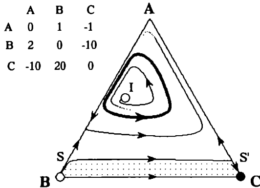
Figure 4. Exemple de jeu avec trois stratégies pures où la sélection naturelle conduit à un cycle limite ou un attracteur ponctuel (•) ; o : point de fuite, S et S' sont des points selle. Dans cet exemple les générations ne se recouvrent pas.
