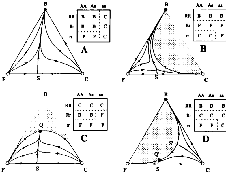
Figure 1. Exemples de dynamique pour le jeu Faucon-Colombe-Bourgeois pour différents déterminismes digéniques des différences entre stratégies (o = point de fuite ; • = attracteur ; S et S' = points-selle). Les zones grisées sont inaccessibles à la population du fait des conditions de panmixie et du déterminisme génétique. Le déterminisme génétique \lambda conduit à une dynamique identique à celle qui prévaut lorsque l'on suppose que chaque stratégie reproduit son propre type.
