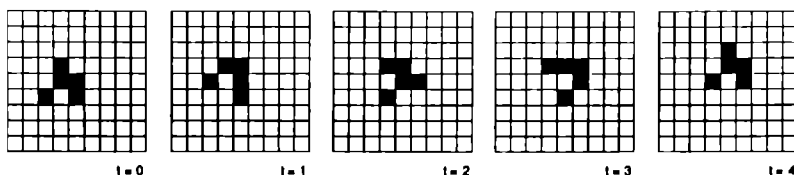
Figure 2. Mouvement d'un glider sur la grille d'un automate cellulaire en dimension 2. Au cours des quatre générations nécessaires au glider pour adopter à nouveau sa forme primitive, la configuration de cellules actives se déplace d'un carré en diagonale.
