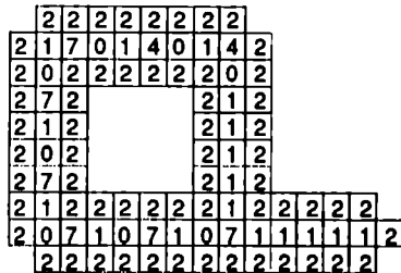
Figure 3. Configuration d'états initiaux caractérisant la structure la plus simple possible capable de s'auto-reproduire.
